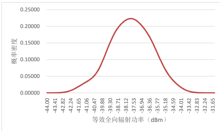
图 A.1 c) 3.5GHz 辐射发射功率检测结果核密度图
