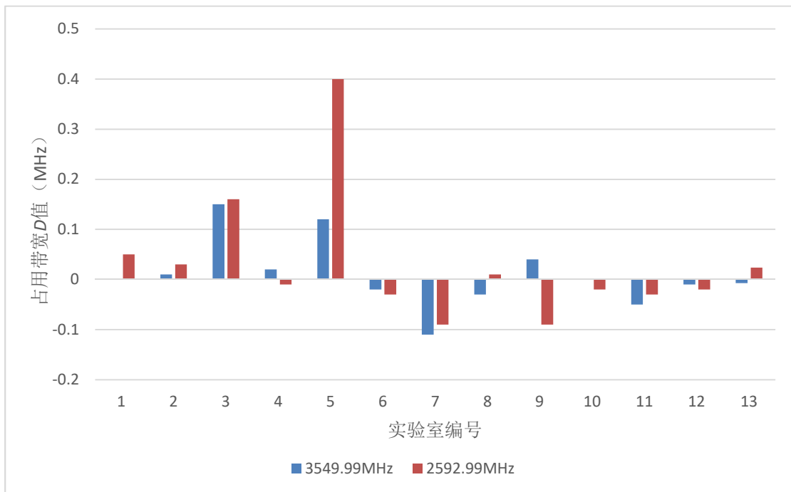
图 B.2 占用带宽检测结果 D 值分布示意图
