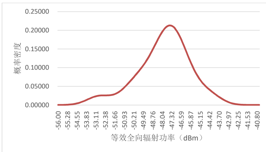
图 A.1 b) 2GHz 辐射发射功率检测结果核密度图
