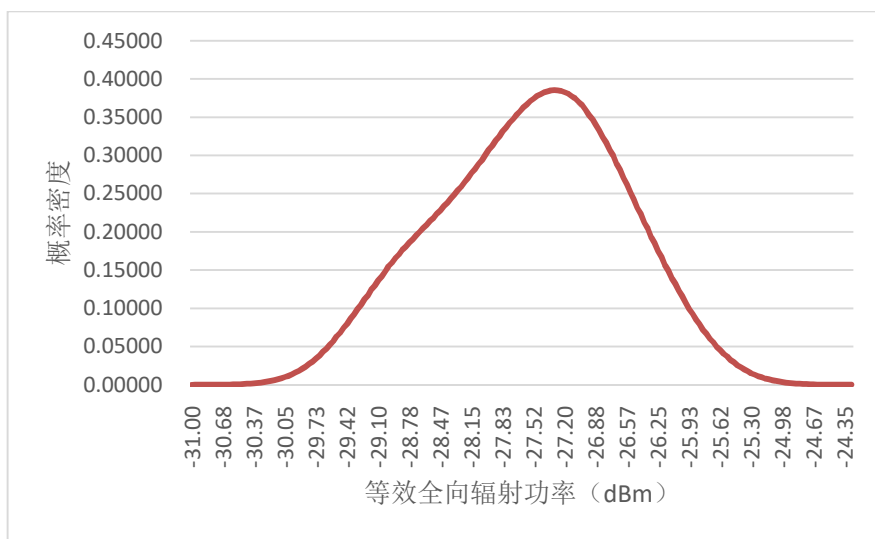
图 A.1 d) 4GHz 辐射发射功率检测结果核密度图
